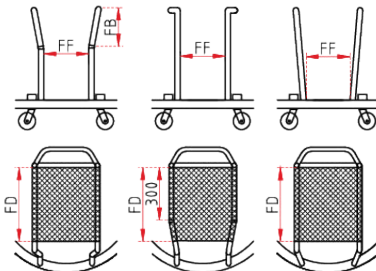
Châssis UV / UV ramme
