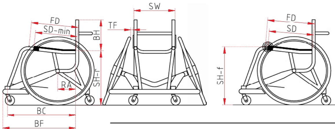
Châssis UV / UV ramme
