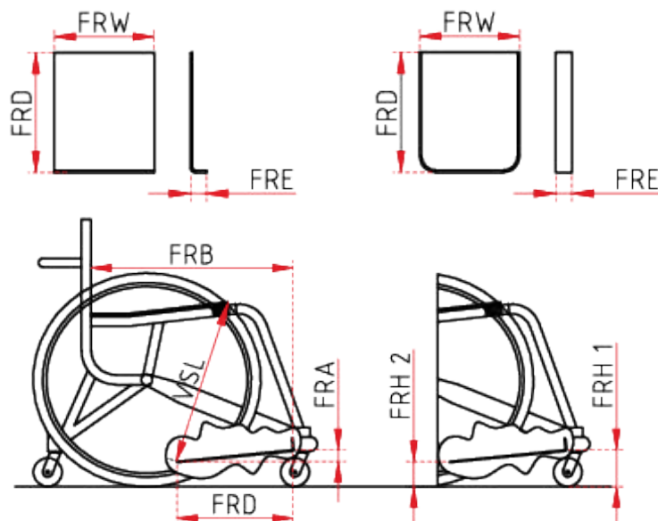
Foot plate (standard) Fodplade (standard)
